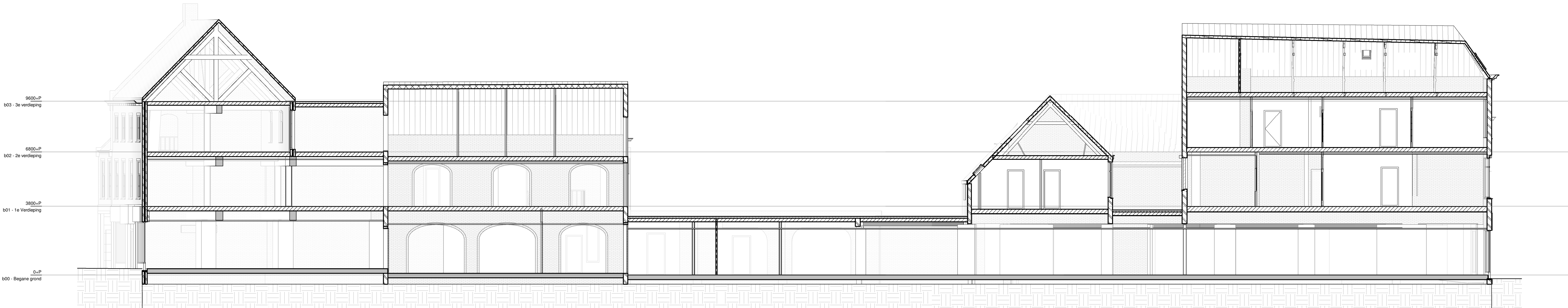
L(22)201, Doorsnede AA1 (bestaand)
