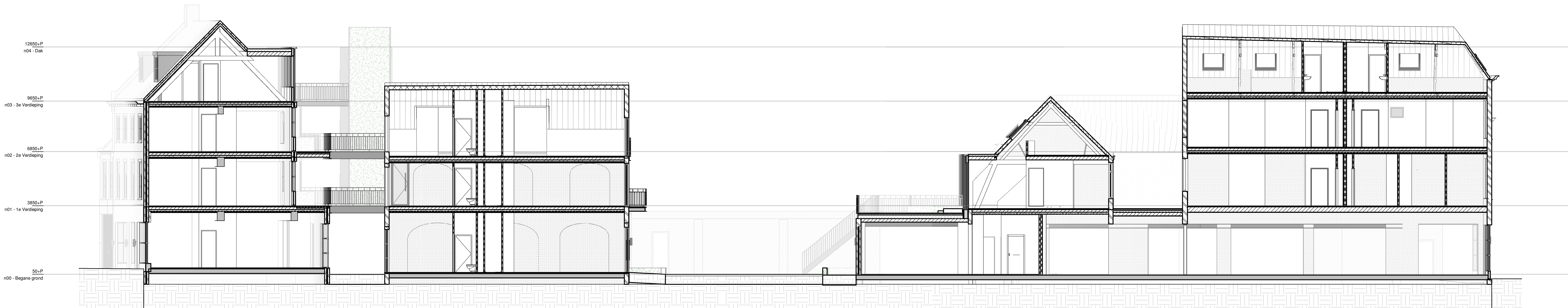
L(22)201, Doorsnede AA1 (nieuw)
