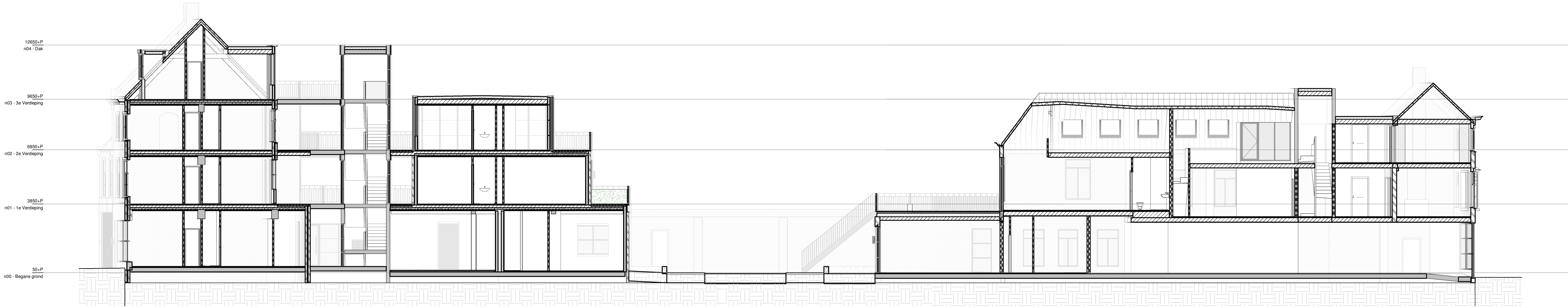
L(22)202, Doorsnede BB1 (nieuw)
