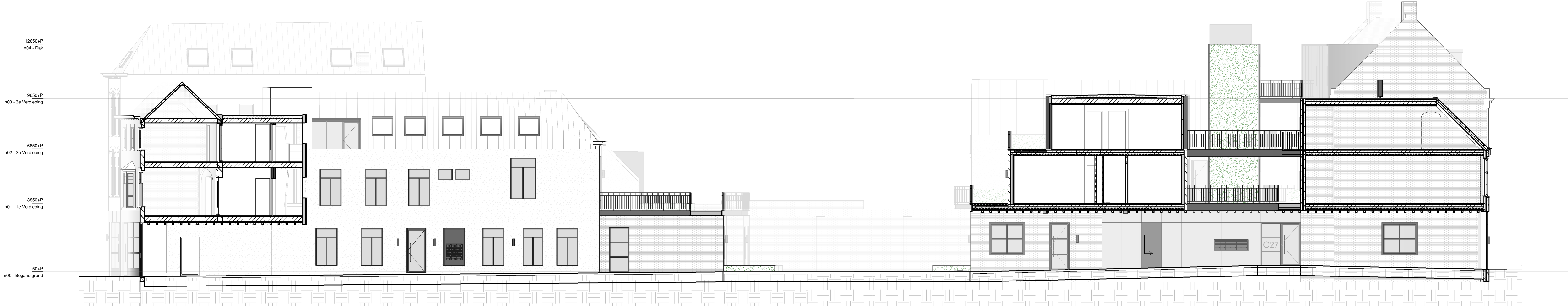
L(22)203, Doorsnede CC2 (nieuw)
